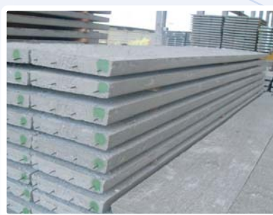
แผ่นพื้น Plank ขนาด 35X5 เซนติเมตร ตามมาตรฐาน มอก. 828-2546
